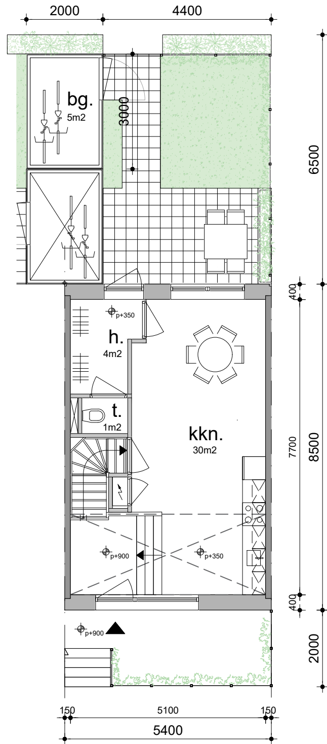
Begane grond BVO 46m 2 GO 39m 2 KAVELOPPERVLAK 89m 2
